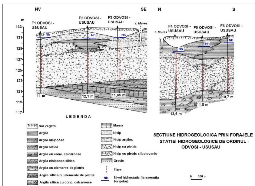
Figura 4.1.1.23 Secțiune hidrogeologică în depozitele aluvionare din lunca și terasele din culoarul Mureșului (zona Odvosi – Ususău)
