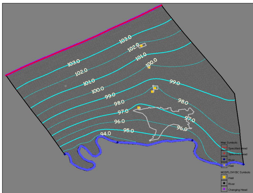
Figura 4.1.1.56 Suprafața piezometrică în cazul introducerii unor captări de 12,5 l/sec
