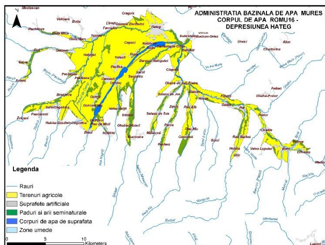
Figura 4.1.1.42 Utilizarea terenului pentru corpul de apă subterană ROMU16 - Depresiunea Hateg
