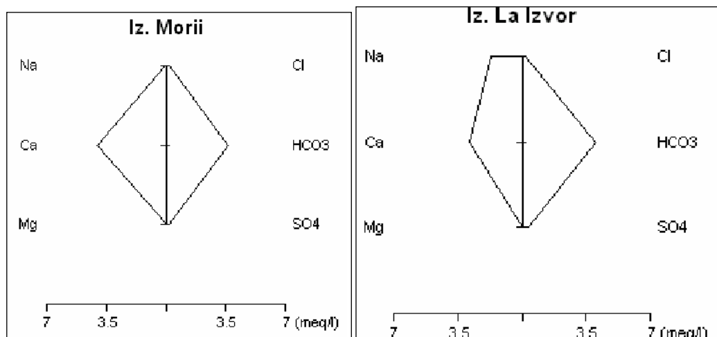
Figura 4.1.1.29 Diagrama Stiff executată pe baza analizelor chimice ale izvoarelor Morii și La Izvor
