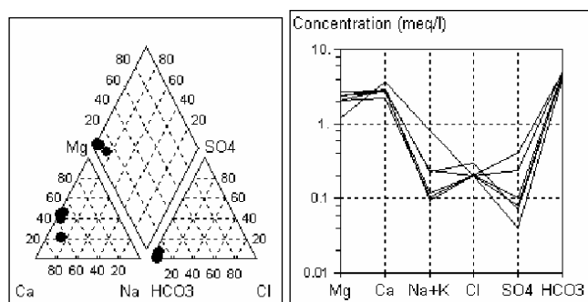
Figura 4.1.1.38 Diagramele Piper și Schoeller efectuate pe baza analizelor chimice a 6 izvoare
