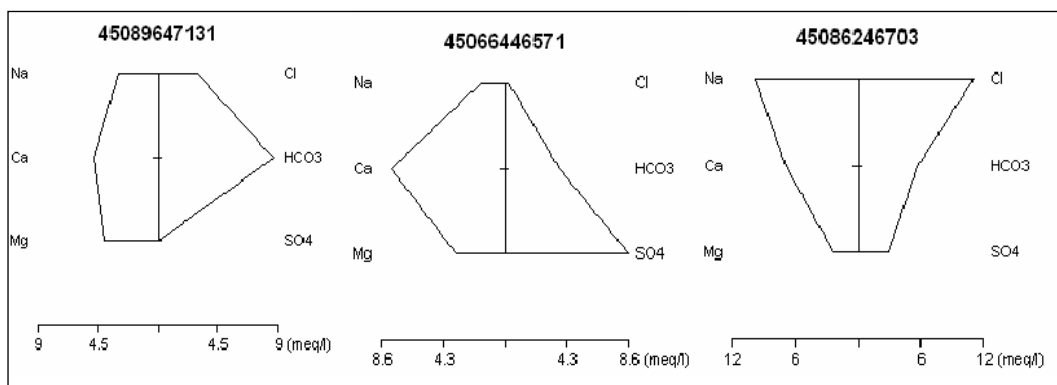
Figura 4.1.1.25 Diagrama Stiff executată pe baza analizelor chimice ale forajelor Miercurea F2, Călan F2 și Orăștie F2
