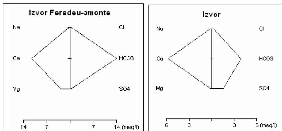
Figura 4.1.1.33 Diagrama Stiff executată pe baza analizelor chimice ale izvoarelor Feredeu și Izvor
