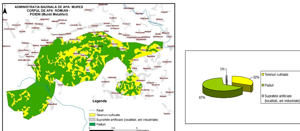
Figura 4.1.1.30 Utilizarea terenului pentru corpul de apă subterană ROMU09 - Poieni
