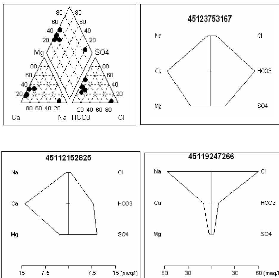
Figura 4.1.1.18 Diagramele Piper și Stiff efectuate pe baza analizelor chimice ale forajelor Copșa Mică F1, F3, Blaj F2, Mediaș F5, Hoghilag F3 și Cristuru-Secuiesc F3
