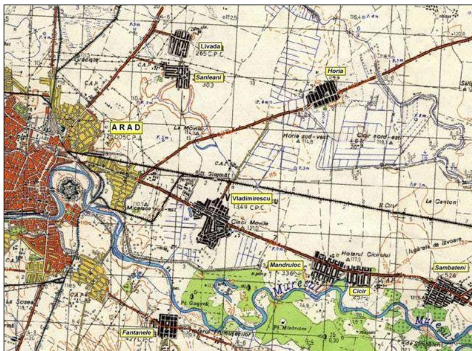
Figura 4.1.1.61 Harta topografică a zonei Cicir
