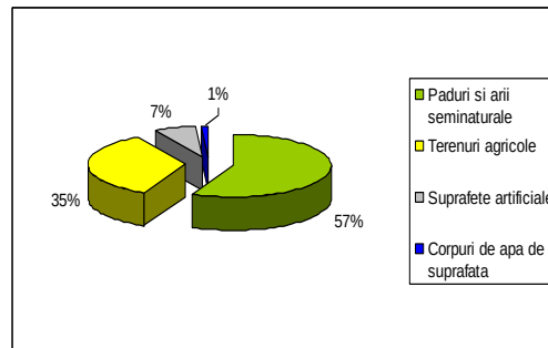
Figura 4.1.1.39 Utilizarea terenului pentru corpul de apă subterană ROMU14 - Lelese
