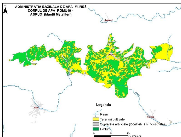
Figura 4.1.1.31 Utilizarea terenului pentru corpul de apă subterană ROMU10 - Abrud
