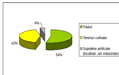
Figura 4.1.1.31 Utilizarea terenului pentru corpul de apă subterană ROMU10 - Abrud
