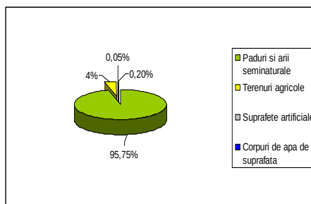
Figura 4.1.1.43 Utilizarea terenului pentru corpul de apă subterană ROMU17- Zeicani
