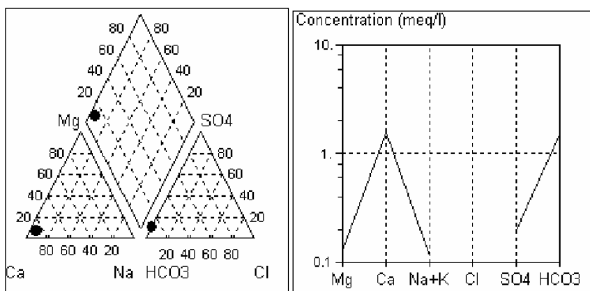
Figura 4.1.1.44 Diagramele Piper și Schoeller efectuate pe baza analizelor chimice ale izvorului de pe pâraul Mucelului
