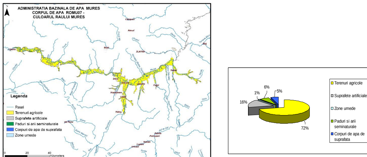
Figura 4.1.1.26 Utilizarea terenului pentru corpul de apă subterană ROMU07- Culoarul râului Mureș
