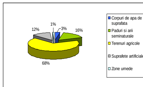
Figura 4.1.1.42 Utilizarea terenului pentru corpul de apă subterană ROMU16 - Depresiunea Hateg
