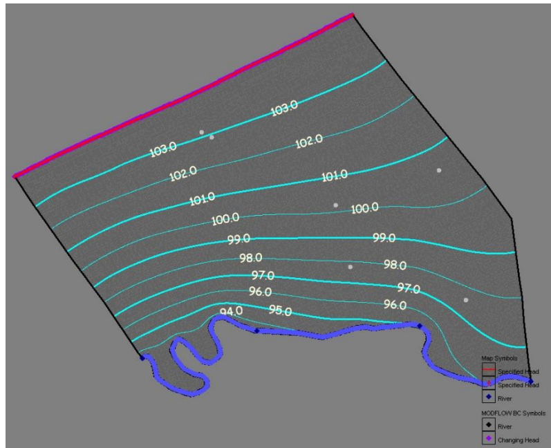
Figura 4.1.1.55 Suprafața piezometrică în cazul reducerii realimentării cu 50%
